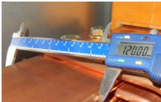
水平母排宽
