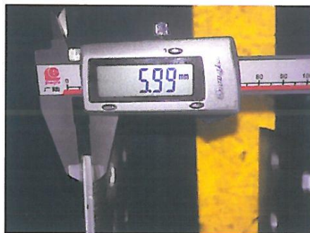
相母排 厚度=6mm
