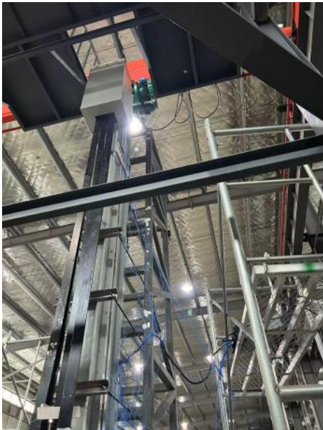
垂直温升试验照片（带分接单元）
