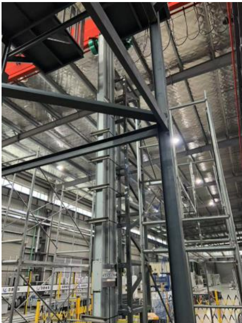
垂直温升试验照片（不带分接单元）
