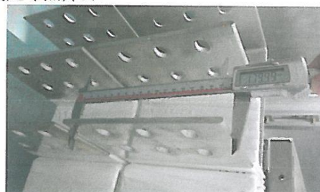
相母排 宽度 180mm (双拼)
