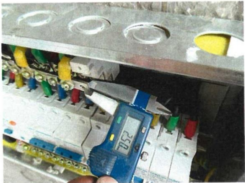
主母线厚
