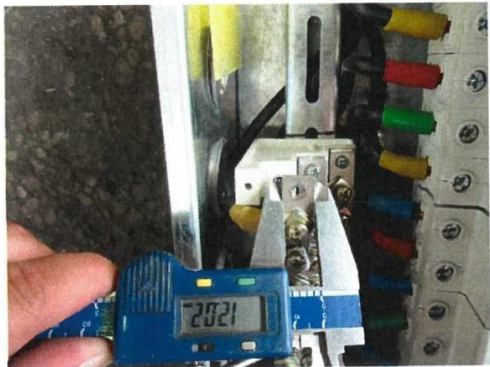
主母线宽
